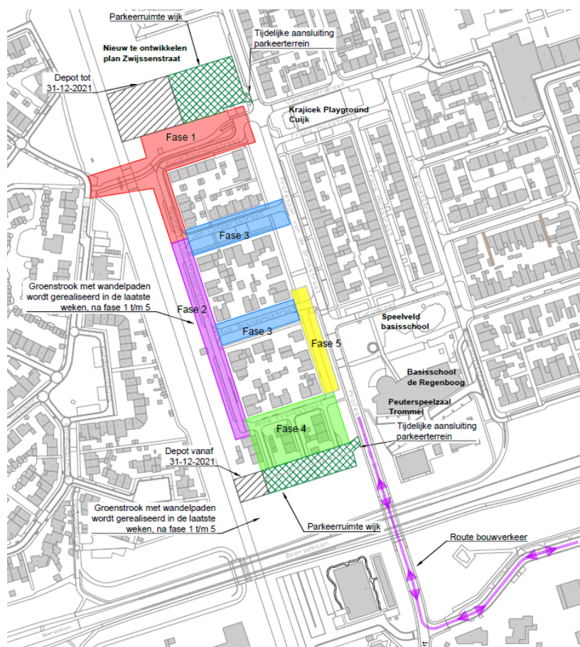
Figuur 1: Faseringstekening
